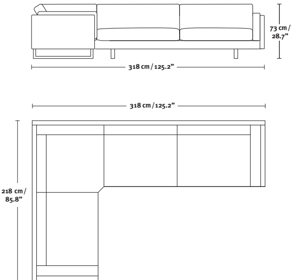
EJ 280-IIR / EJ 280-IIL
